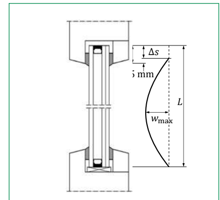
Bild 7: Sehnverkürzung \Delta s , maximale Durchbiegung w_{\max} , Bezugslänge L und verbleibender Glaseinstand i - \Delta s \geq 5 mm, hier gezeigt an der Oberkante eines Isolierglases
