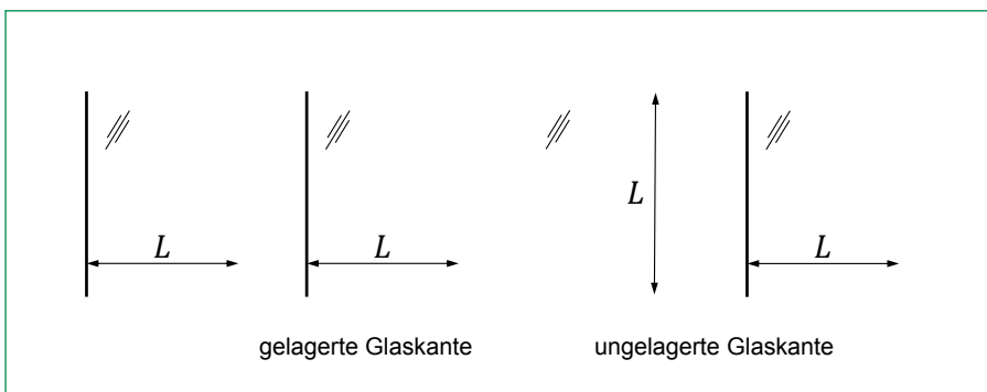
Bild 5: Stützweite als Bezugslänge L von vier-, drei- und zweiseitig linienförmig gelagerten Rechteckscheiben
