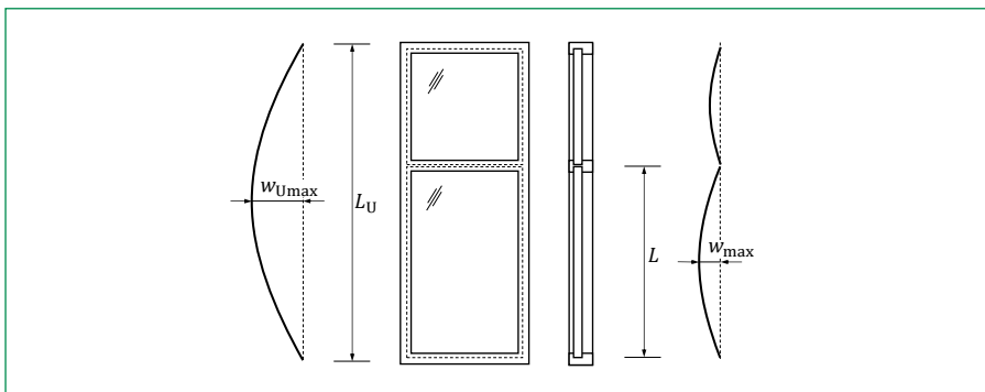
Bild 4: Bezugslänge L der aufgelagerten Scheiben im Vergleich zur Länge der Unterkonstruktion L_U
