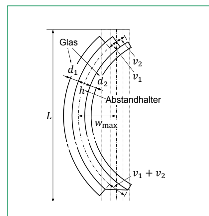
Bild 8: Verschiebungen v_j zwischen Glas und Abstandhalter (oben) sowie Verschiebung der Glaskanten (unten) im Randbereich einer durchgebogenen Isolierglaskante
